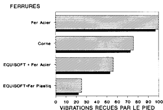
Figure 5 : Comparaison de l'amortissement procuré par différentes ferrures.
